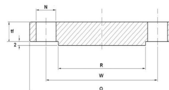
CEGO Blind
